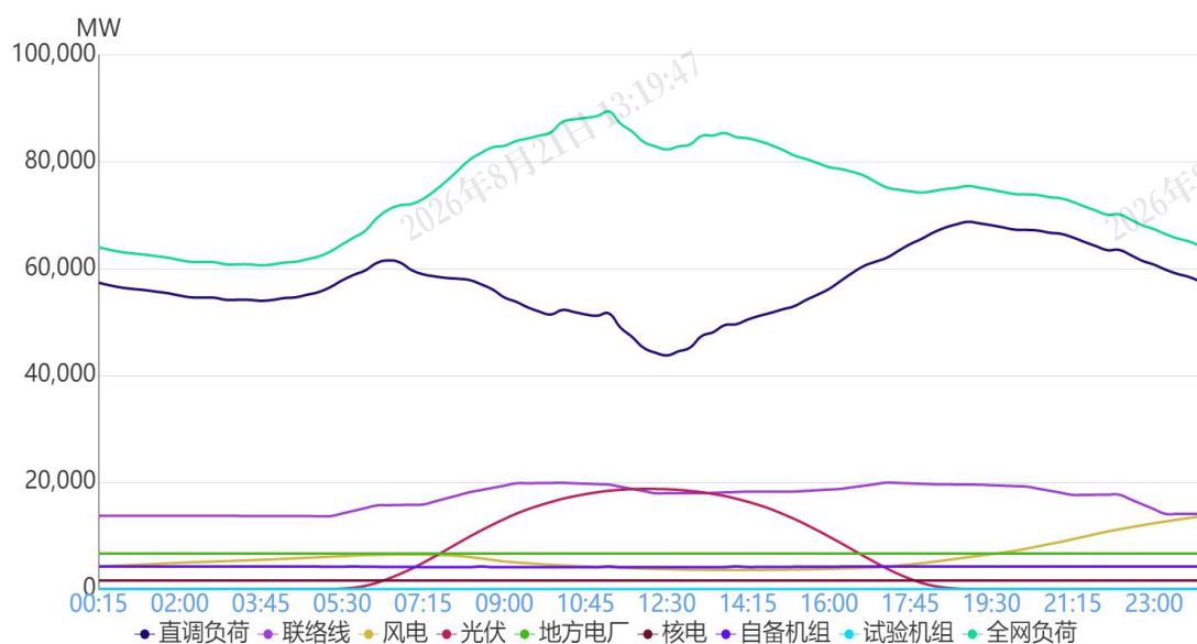
图 1 4月23日负荷及电源出力预测情况
