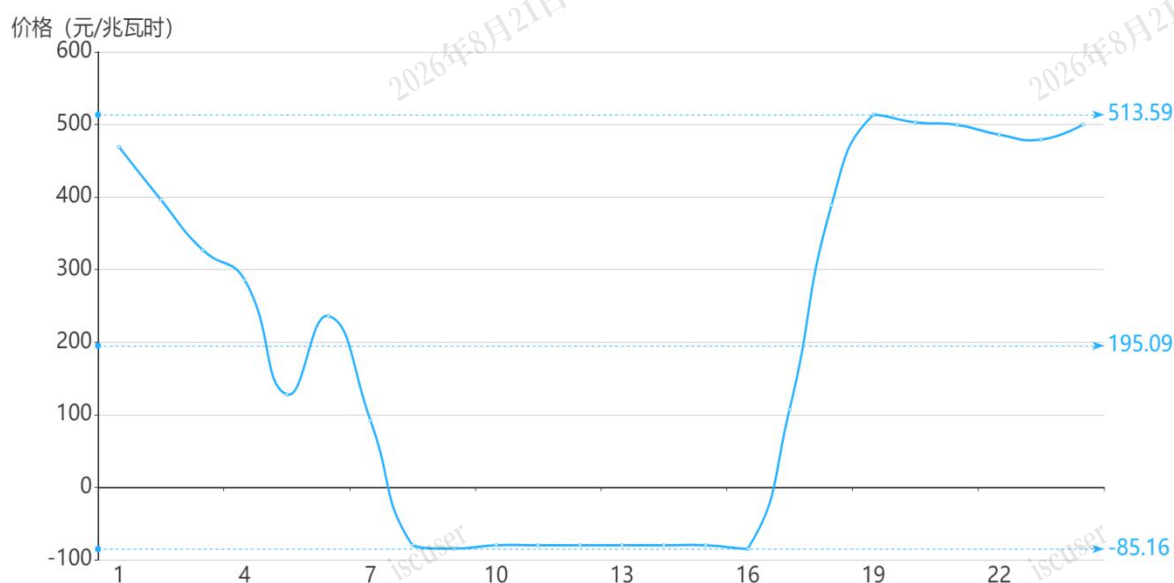
图3 4月22日实时市场用电侧价格
