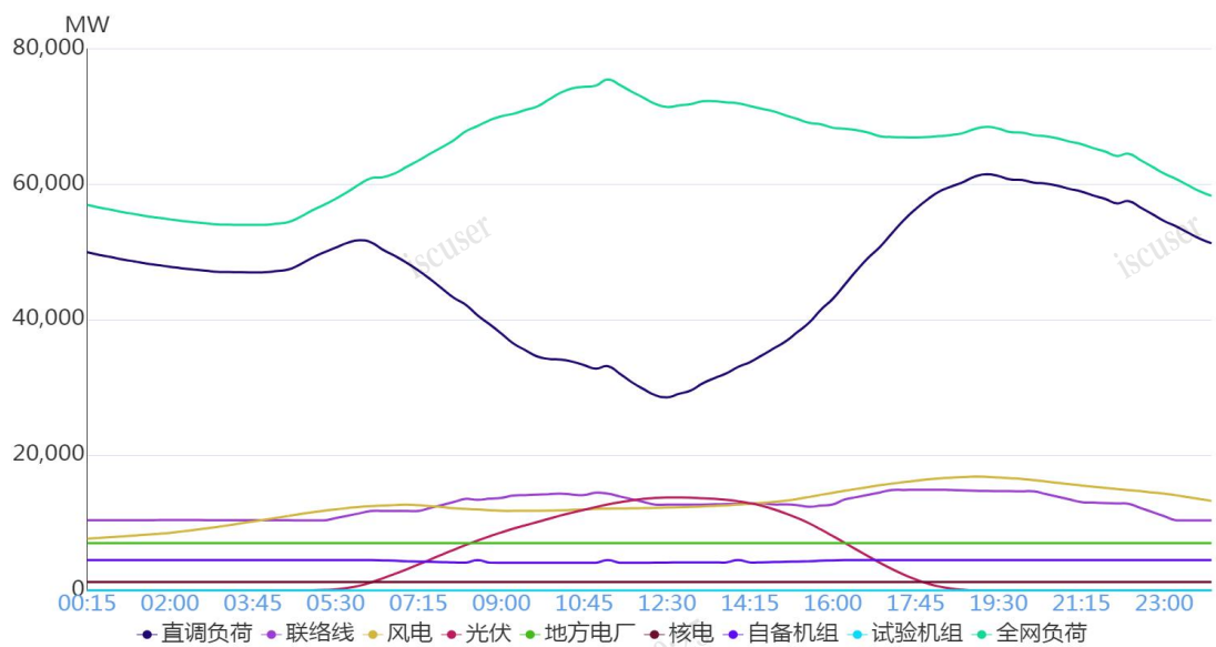
图 1 5 月 2 日负荷及电源出力预测情况
