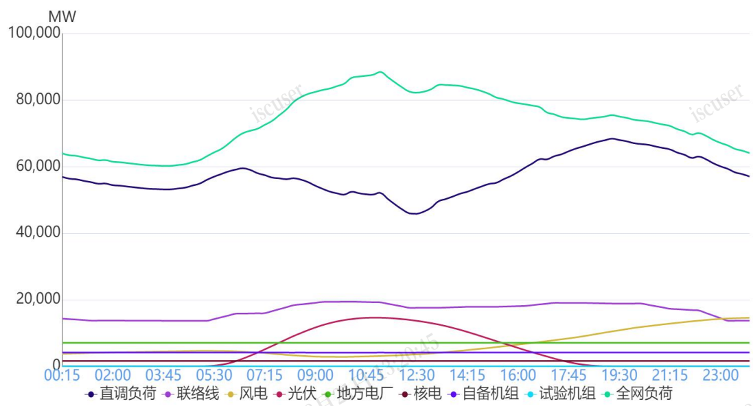
图 1 5月7日负荷及电源出力预测情况
