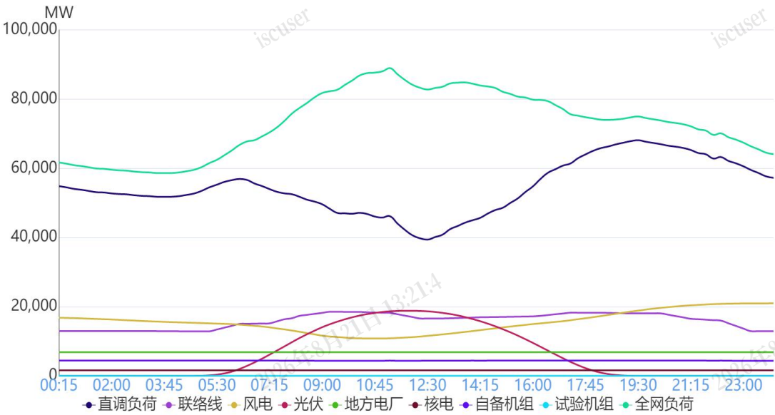
图1 5月12日负荷及电源出力预测情况
