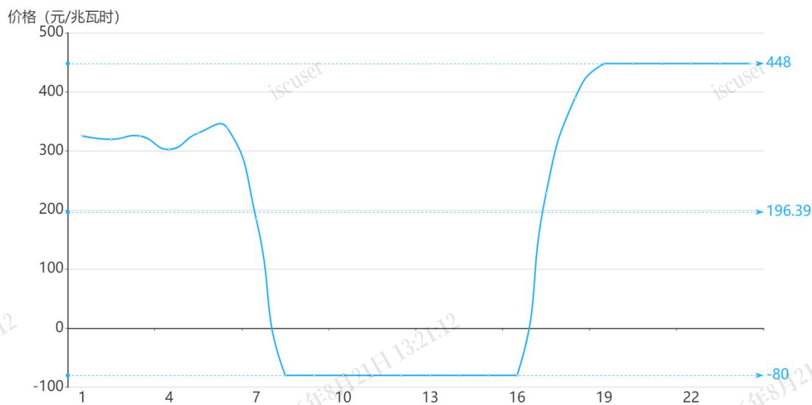
图2 5月14日日前市场用电侧价格
