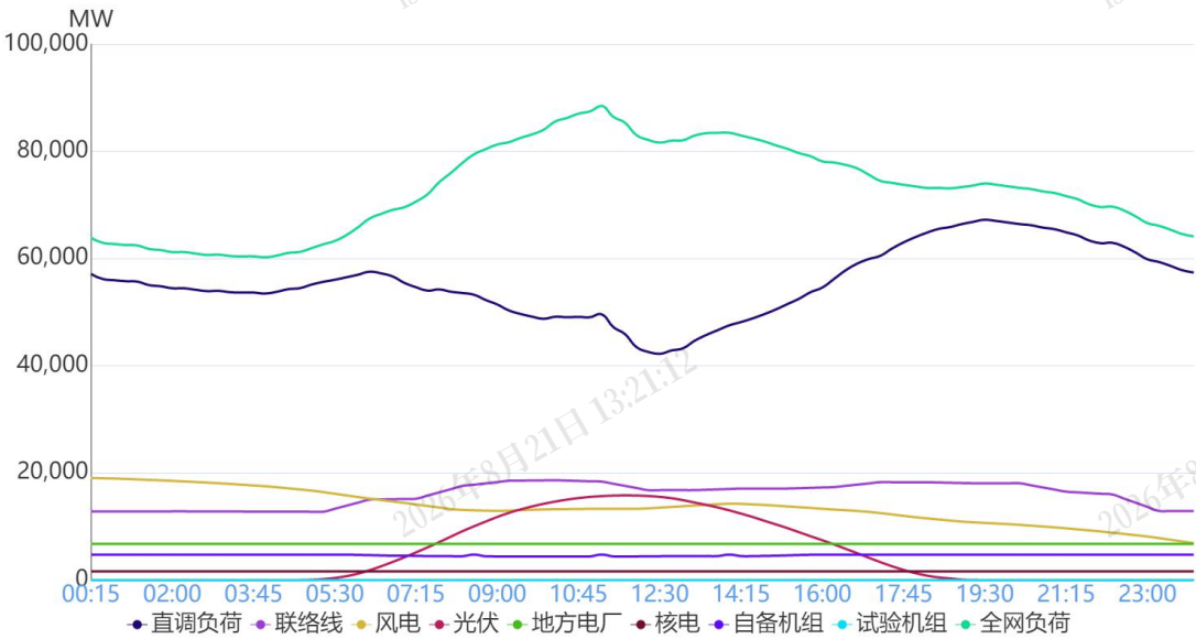
图1 5月14日负荷及电源出力预测情况
