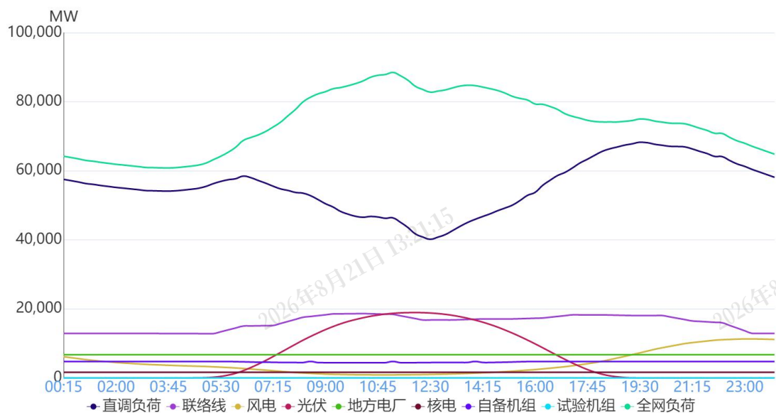
图1 5月15日负荷及电源出力预测情况
