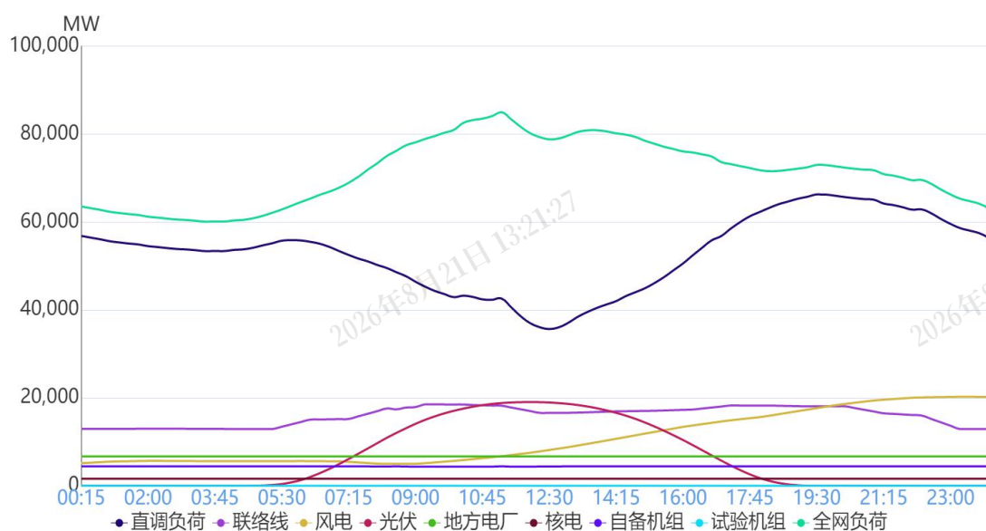
图 1 5月18日负荷及电源出力预测情况
