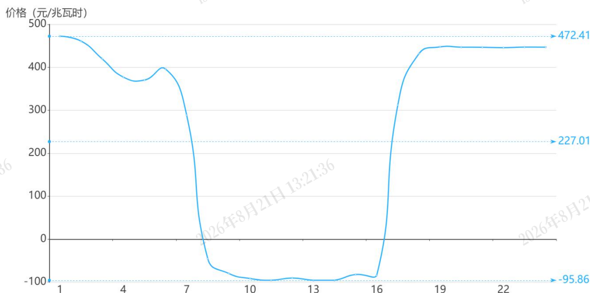
图2 5月20日日前市场用电侧价格
