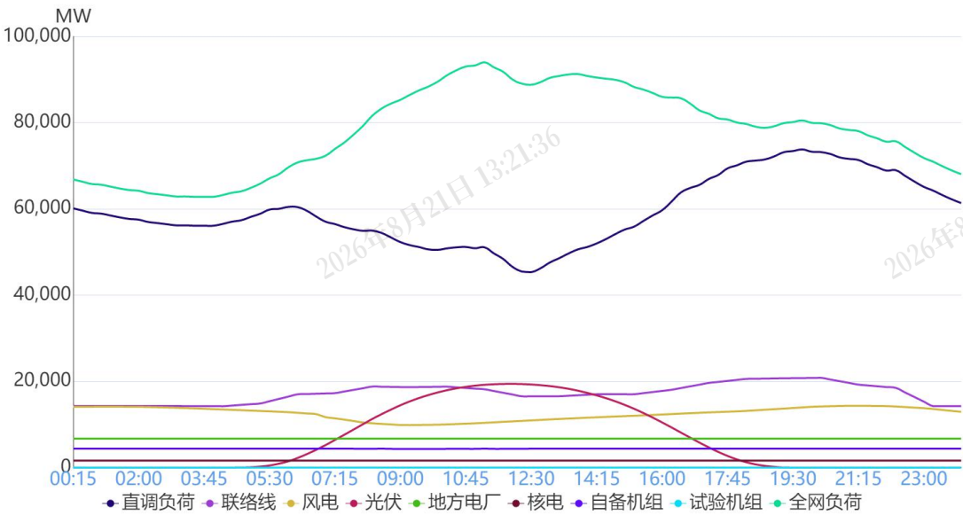
图1 5月20日负荷及电源出力预测情况
