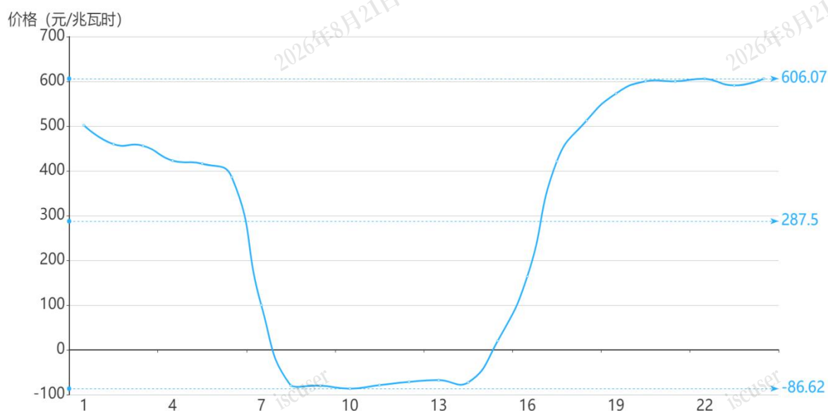
图3 5月25日实时市场用电侧价格
