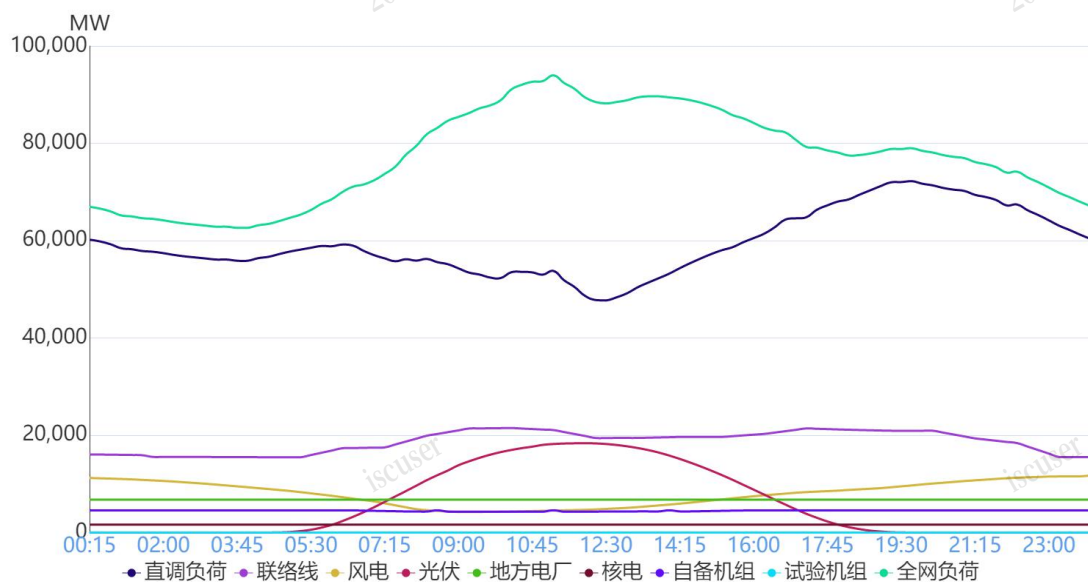
图 1 5月30日负荷及电源出力预测情况
