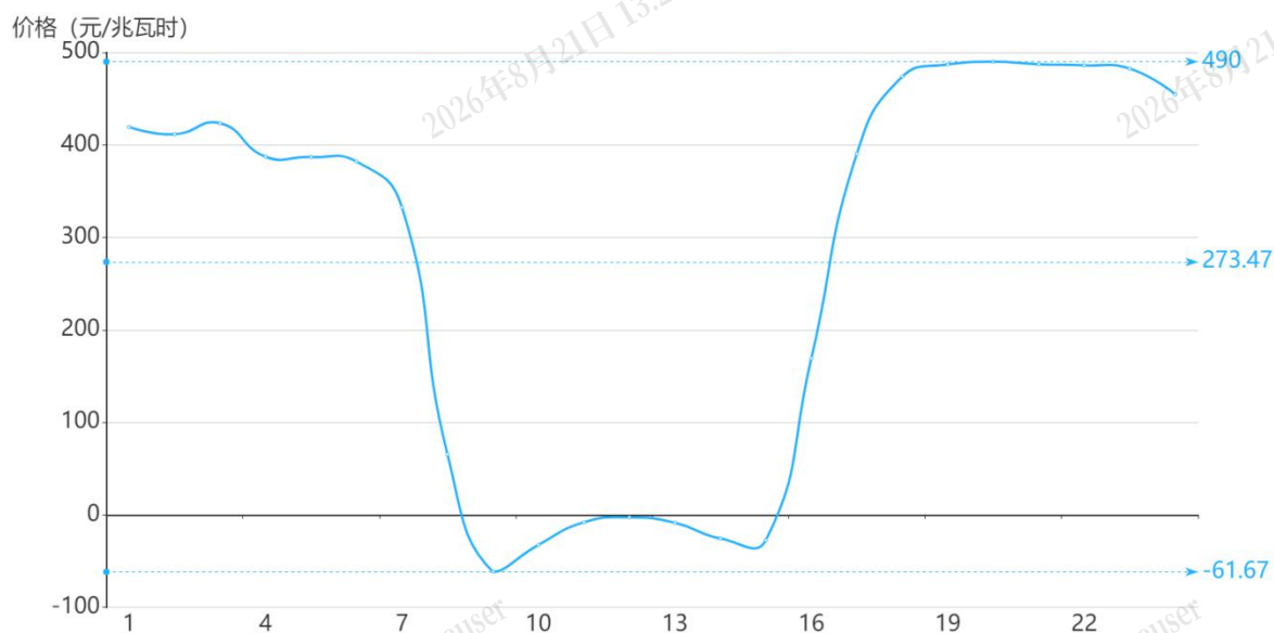
图 2 5 月 30 日日前市场用电侧价格
