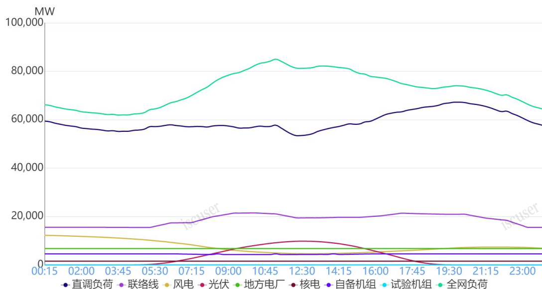
图1 5月31日负荷及电源出力预测情况
