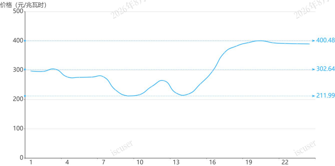
图 2 5 月 31 日日前市场用电侧价格
