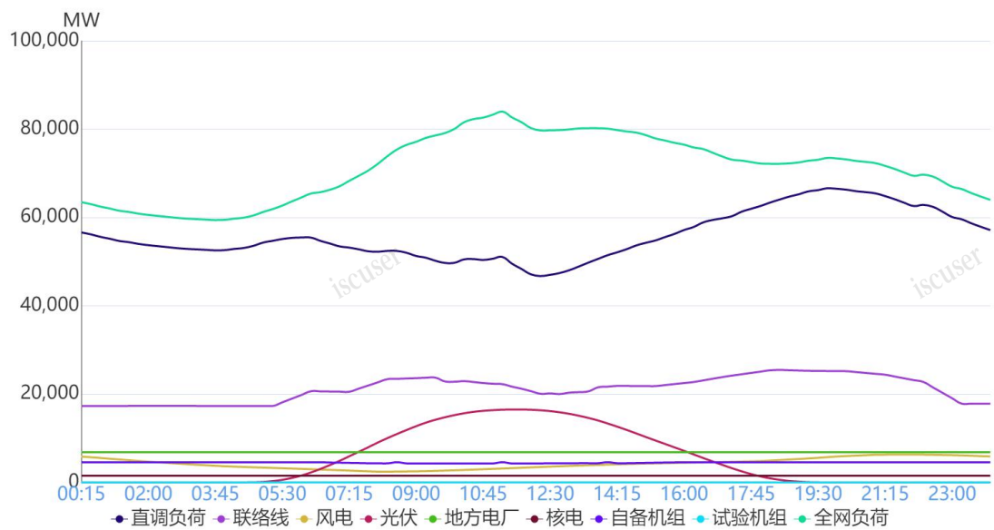
图 1 6 月 1 日负荷及电源出力预测情况
