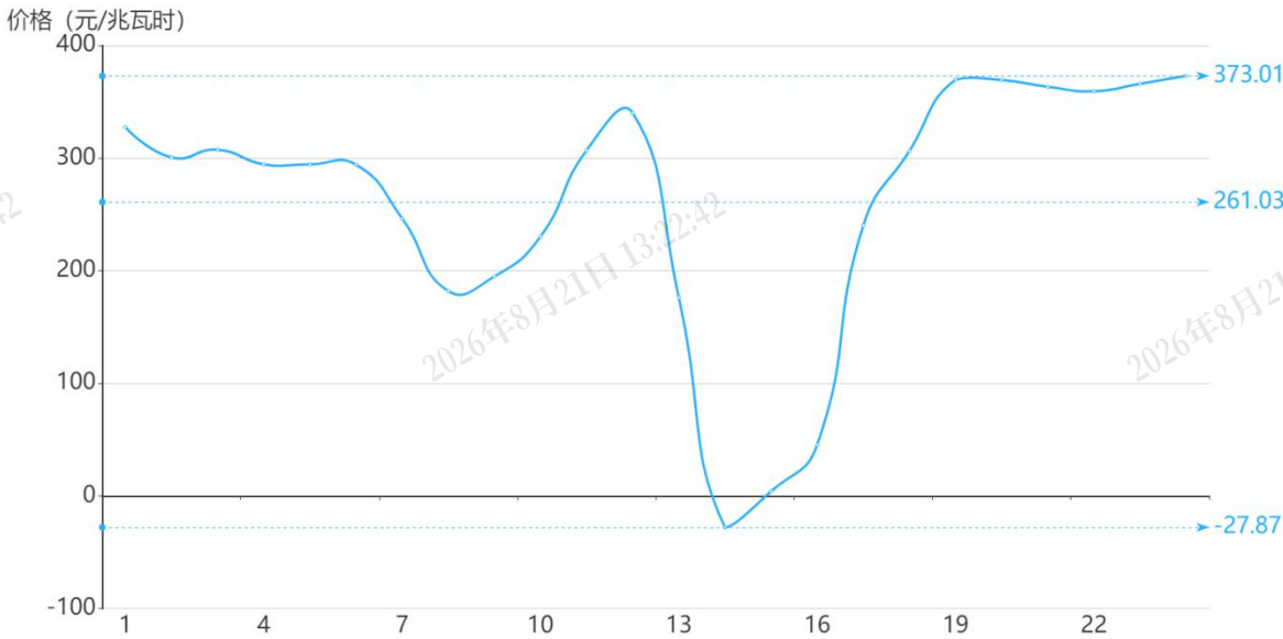
图3 5月31日实时市场用电侧价格
