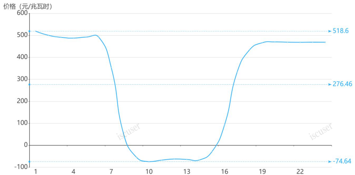
图2 6月1日日前市场用电侧价格
