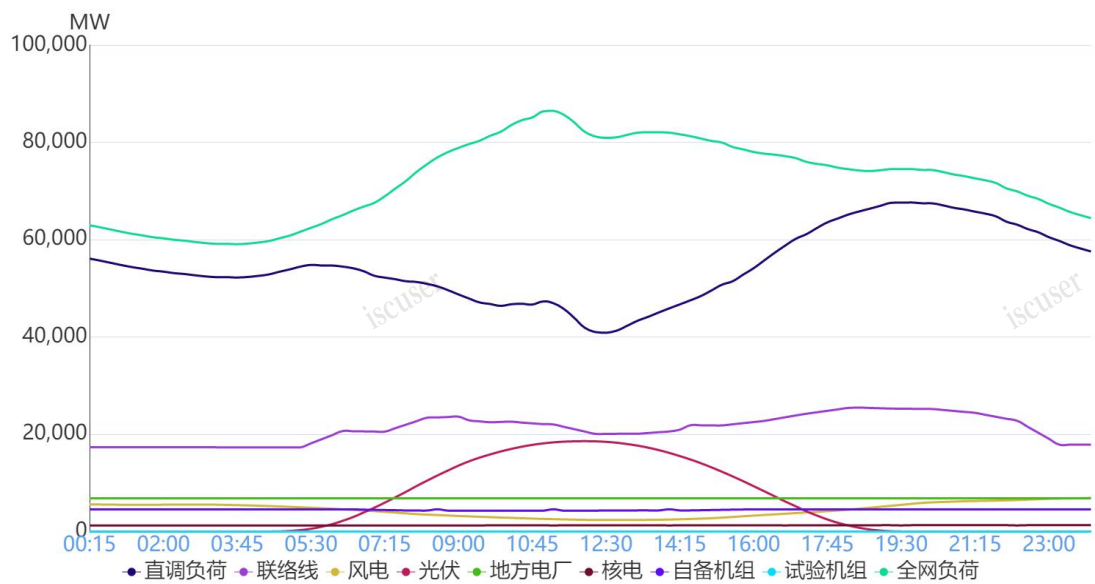
图 1 6 月 2 日负荷及电源出力预测情况
