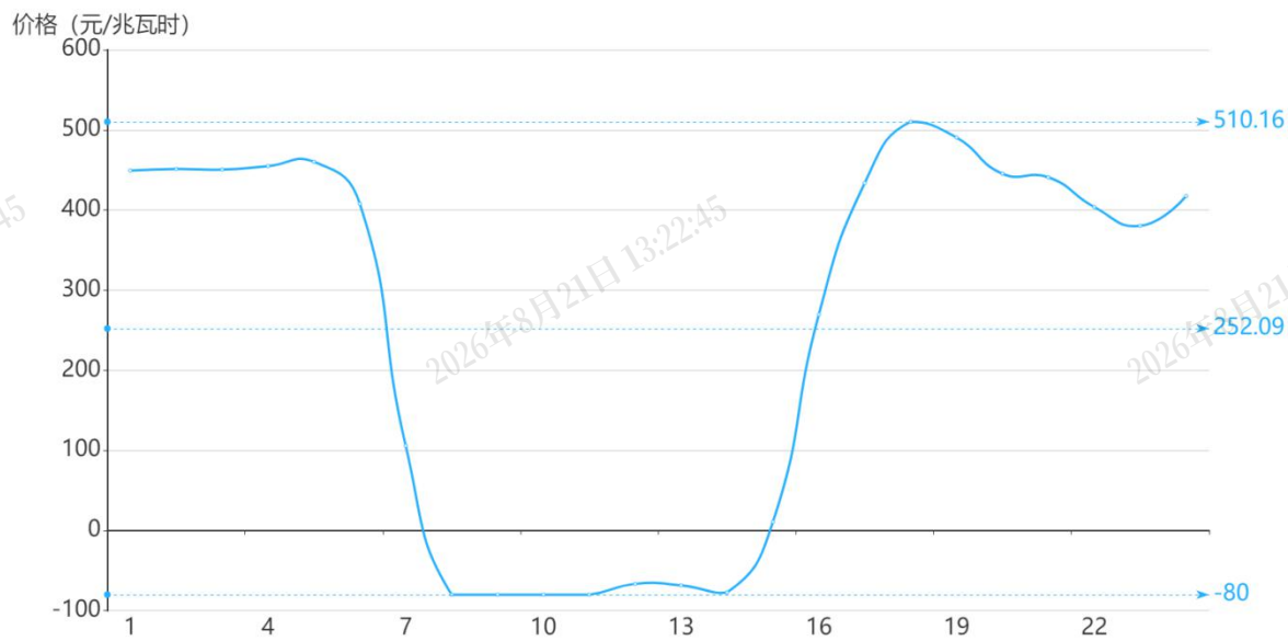
图3 6月1日实时市场用电侧价格
