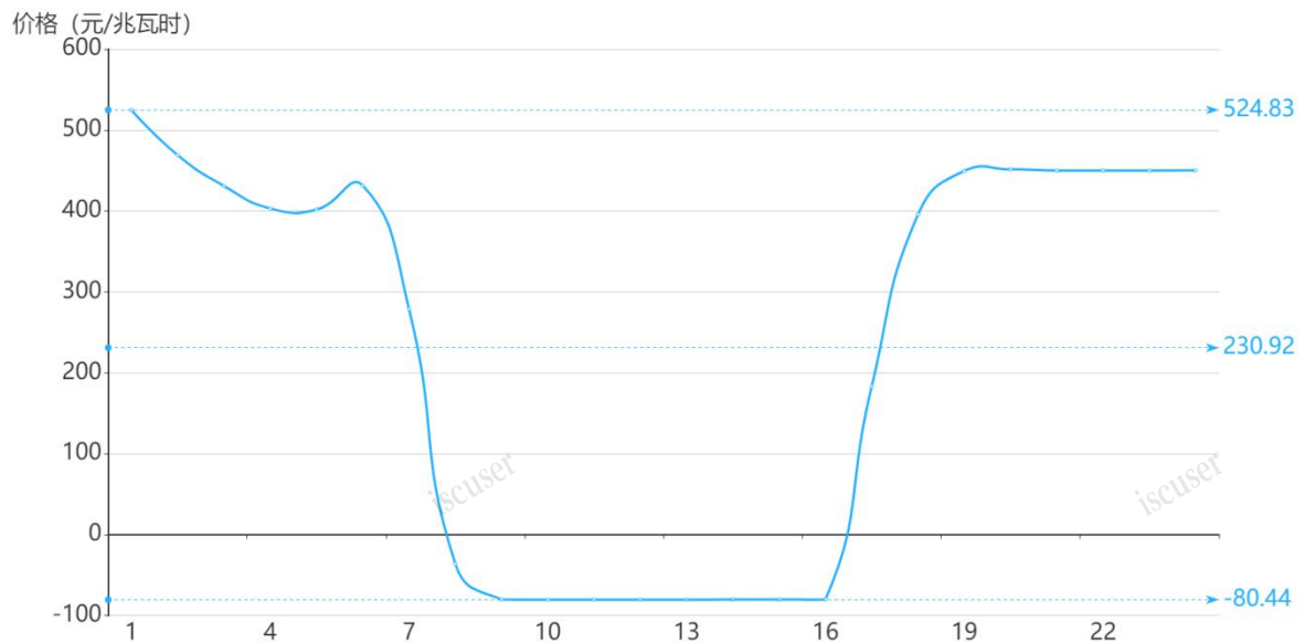
图 2 6 月 2 日日前市场用电侧价格
