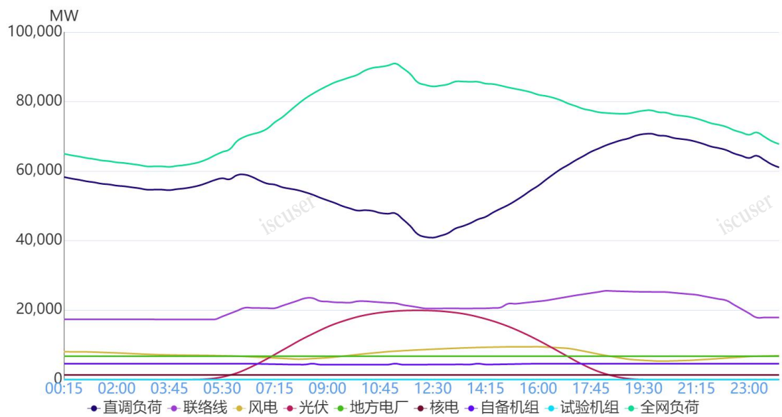
图 1 6 月 3 日负荷及电源出力预测情况
