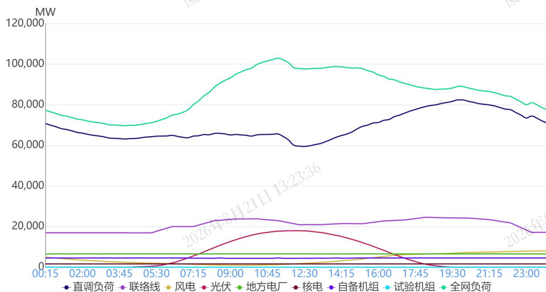
图 1 6月14日负荷及电源出力预测情况
