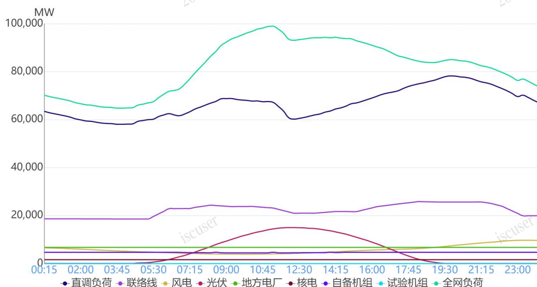
图 1 6月30日负荷及电源出力预测情况
