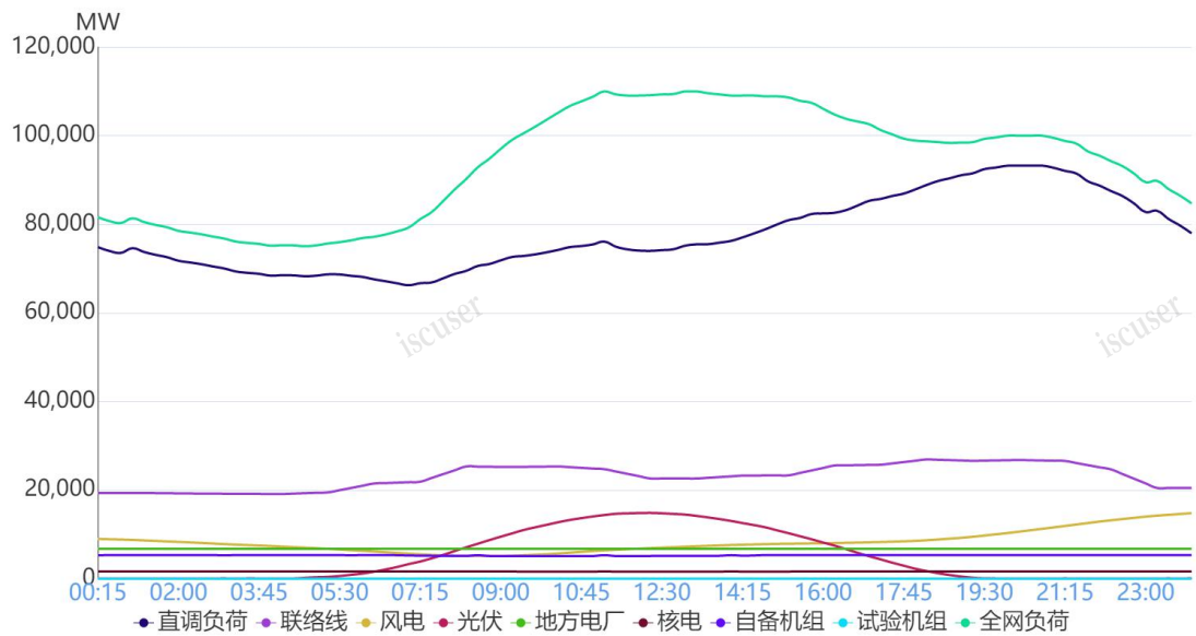
图 1 7 月 2 日负荷及电源出力预测情况
