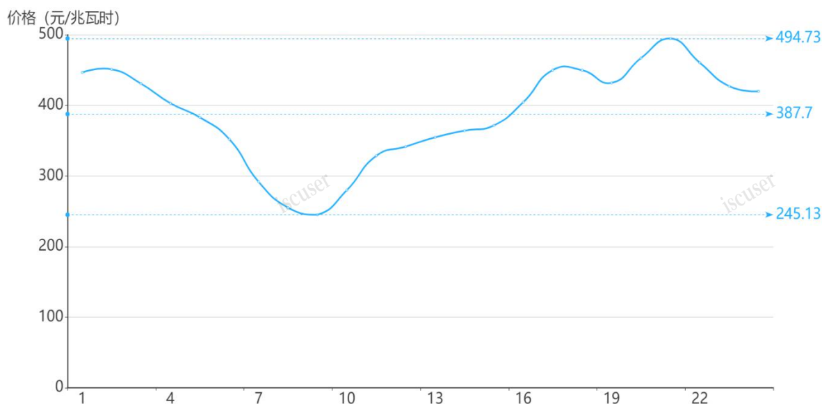
图2 7月7日日前市场用电侧价格
