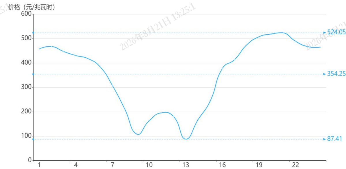
图 3 7 月 6 日实时市场用电侧价格
