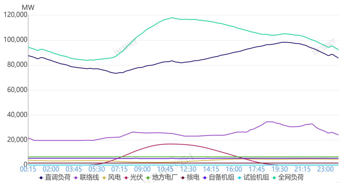
图 1 7月7日负荷及电源出力预测情况
