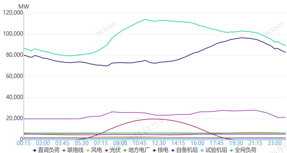
图 1 7月9日负荷及电源出力预测情况
