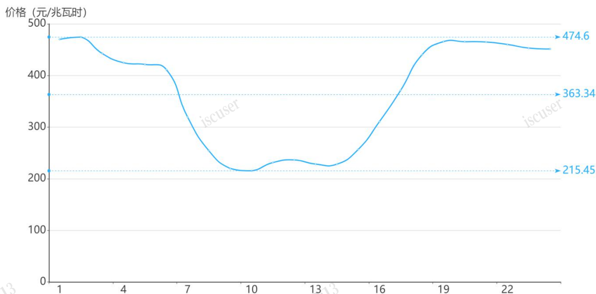
图2 7月10日日前市场用电侧价格
