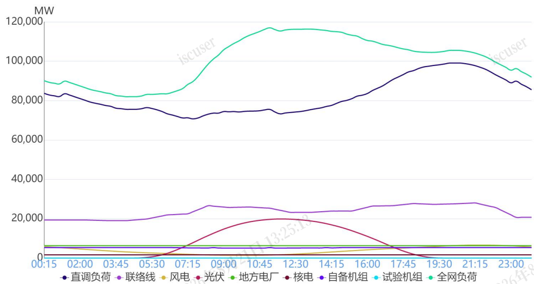
图 1 7月10日负荷及电源出力预测情况
