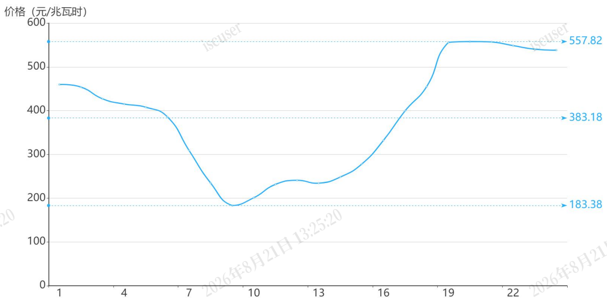
图2 7月12日日前市场用电侧价格
