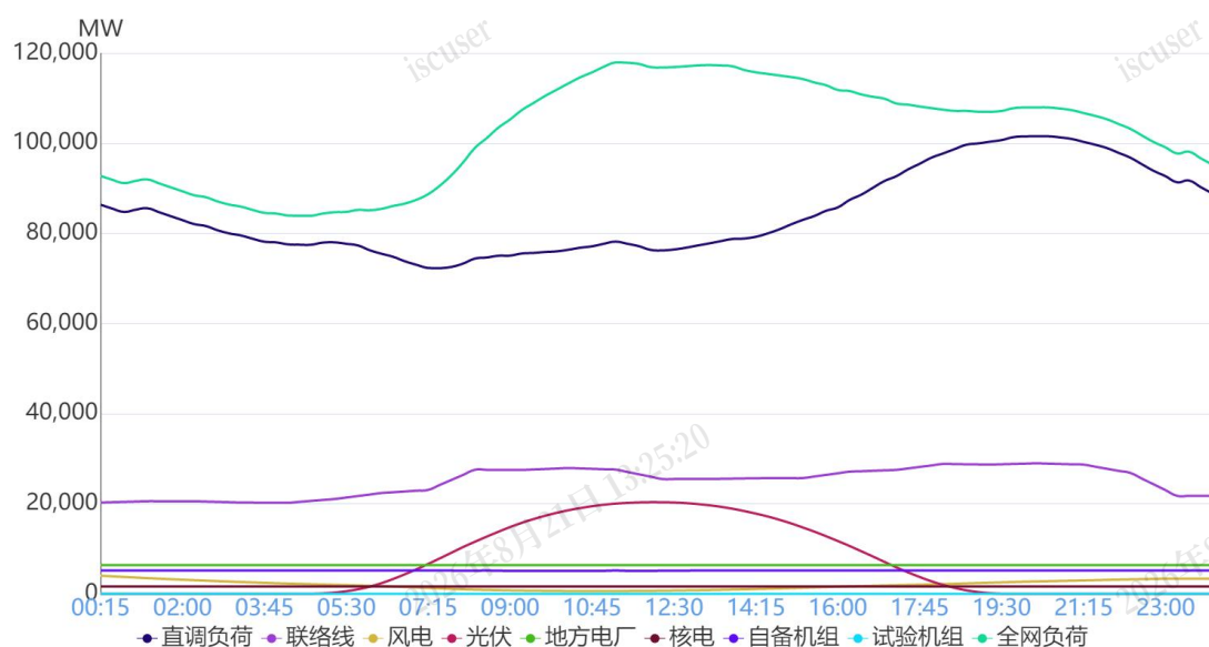
图 1 7月12日负荷及电源出力预测情况
