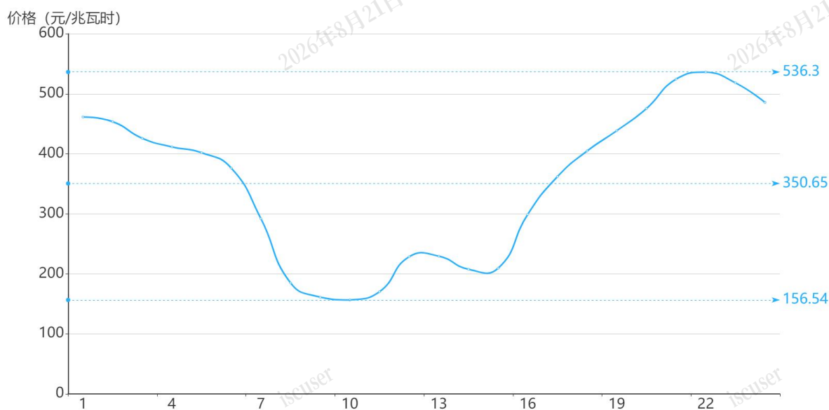
图3 7月11日实时市场用电侧价格
