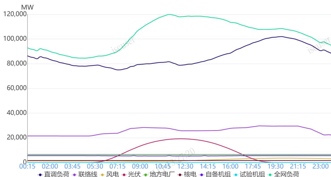
图 1 8月7日负荷及电源出力预测情况
