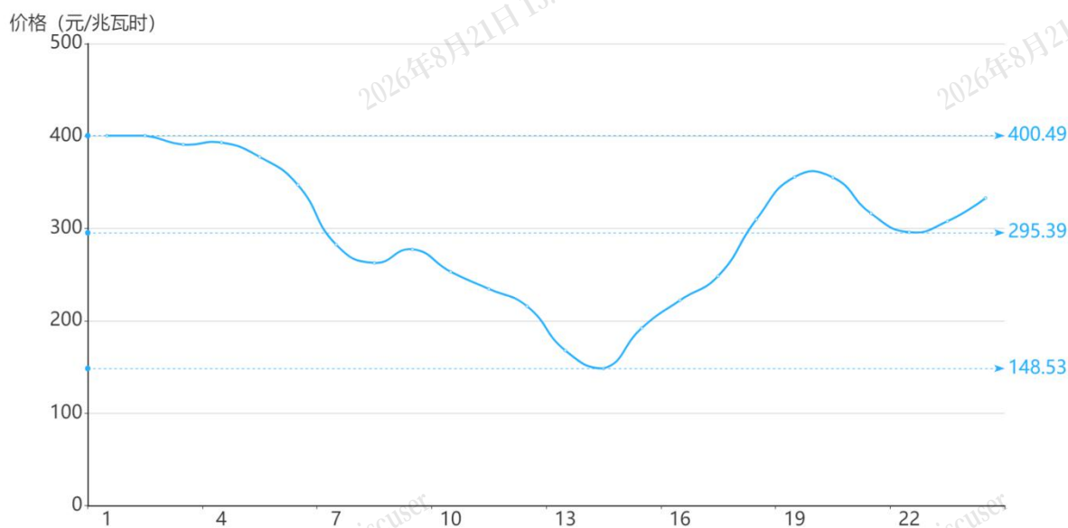
图 3 8 月 9 日实时市场用电侧价格
