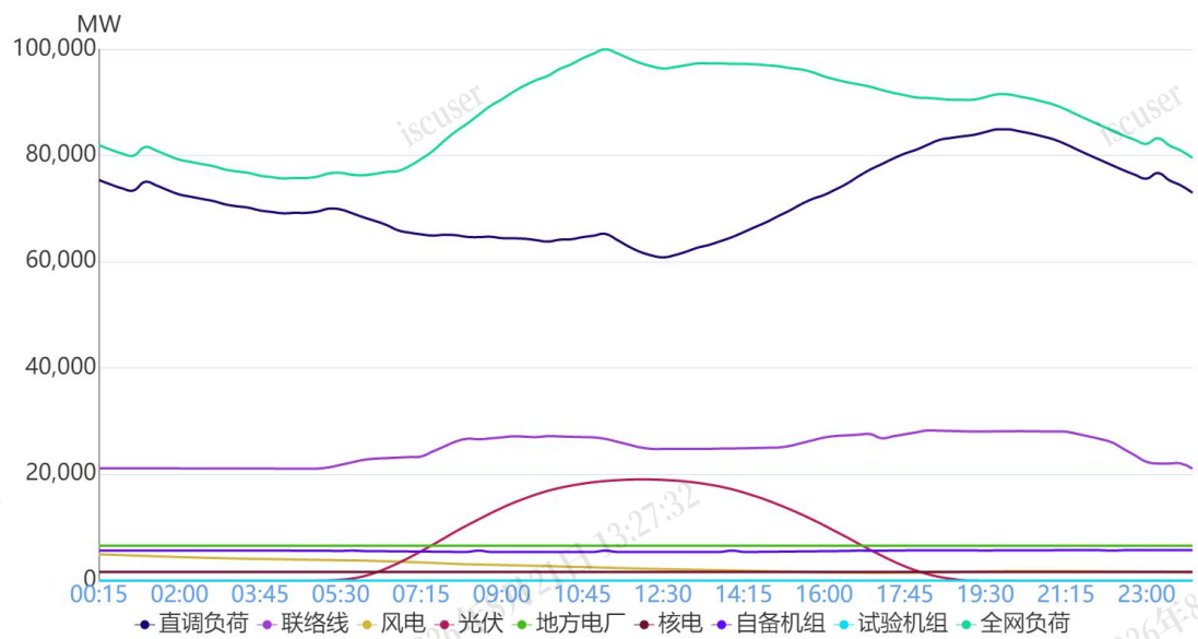
图 1 8月10日负荷及电源出力预测情况
