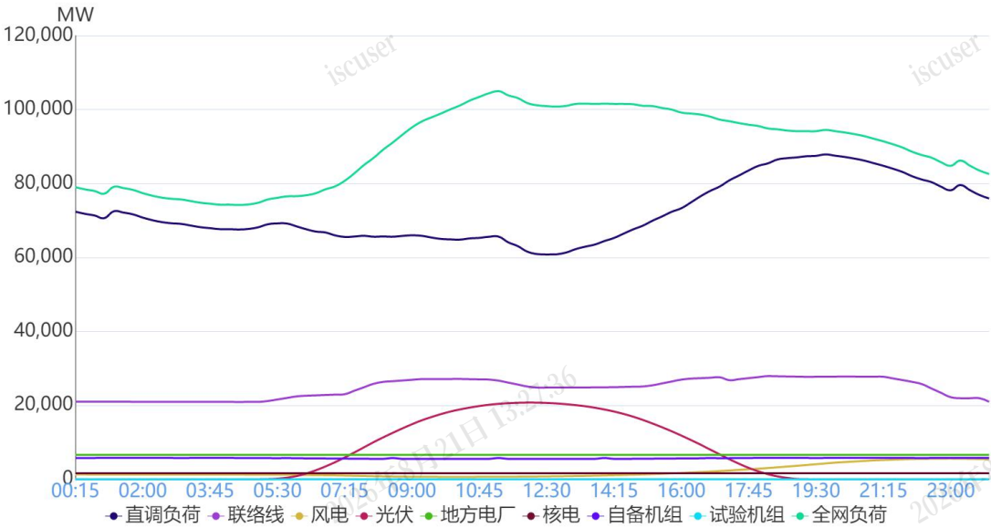
图 1 8月11日负荷及电源出力预测情况
