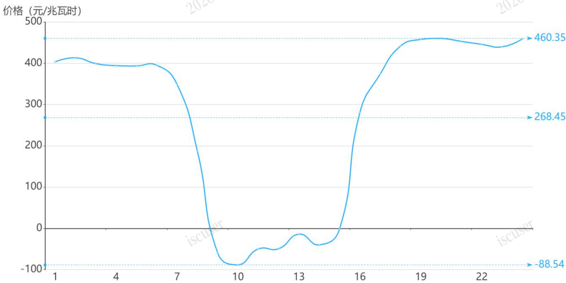
图 3 8 月 10 日实时市场用电侧价格
