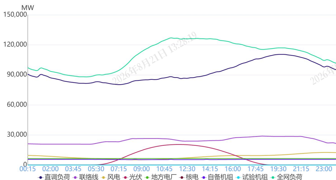
图 1 8月21日负荷及电源出力预测情况
