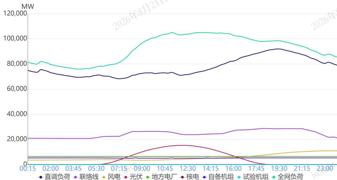
图 1 8月27日负荷及电源出力预测情况
