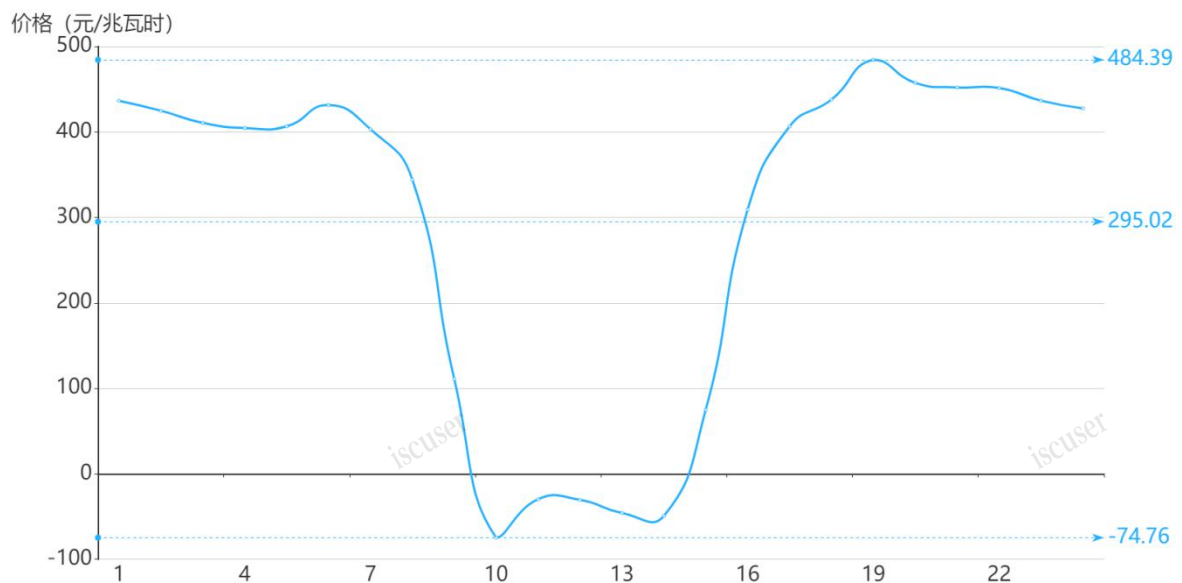
图2 9月1日日前市场用电侧价格
