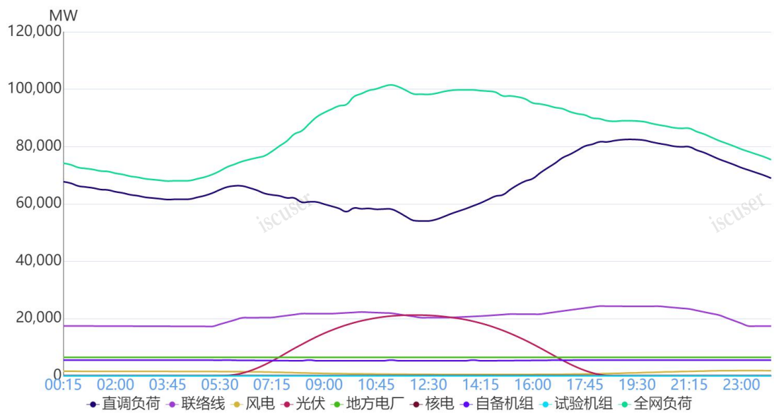
图 1 9 月 1 日负荷及电源出力预测情况
