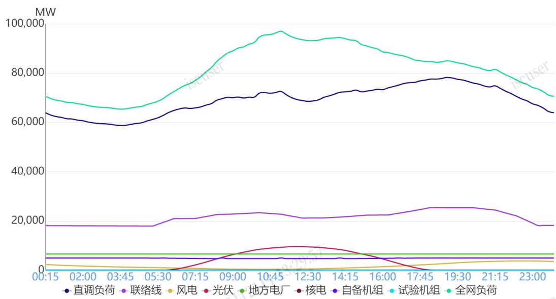
图 1 9月8日负荷及电源出力预测情况
