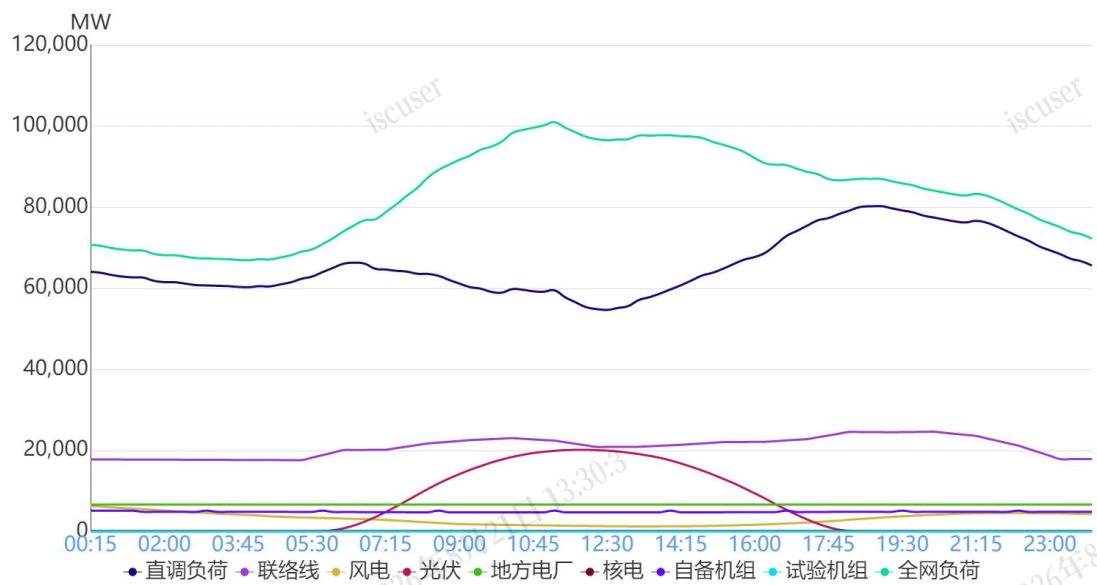
图 1 9月10日负荷及电源出力预测情况
