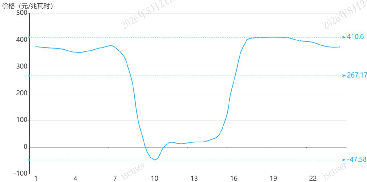
图 3 9 月 9 日实时市场用电侧价格
