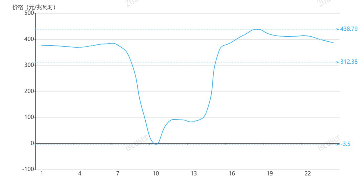
图 3 9 月 10 日实时市场用电侧价格
