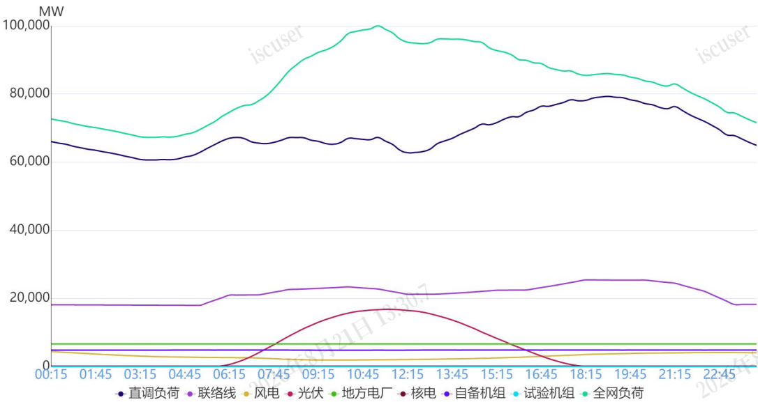
图 1 9月11日负荷及电源出力预测情况
