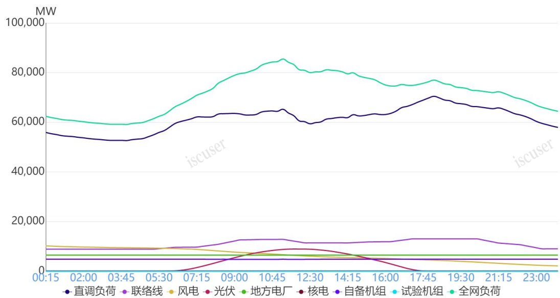
图 1 10 月 3 日负荷及电源出力预测情况
