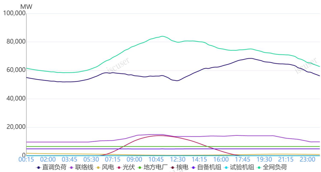
图 1 10 月 4 日负荷及电源出力预测情况
