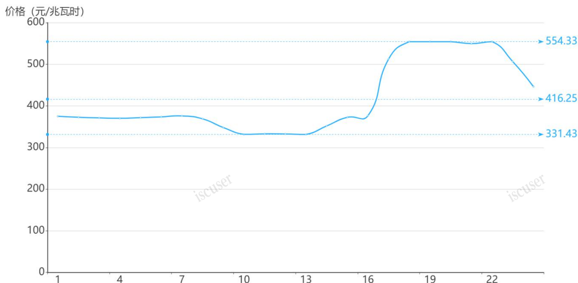
图2 10月4日日前市场用电侧价格
