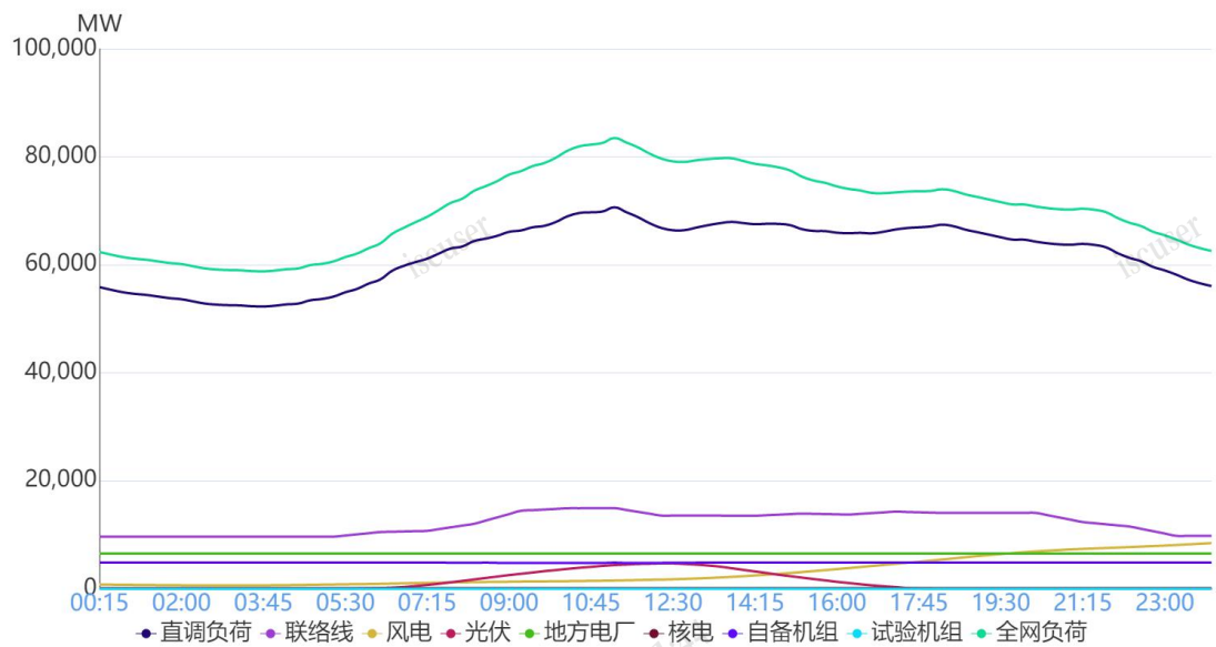
图 1 10 月 5 日负荷及电源出力预测情况
