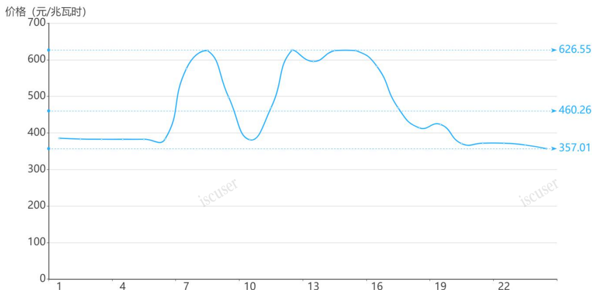
图2 10月5日日前市场用电侧价格
