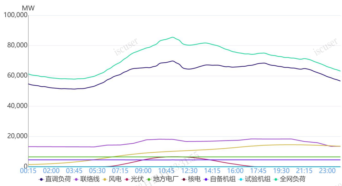
图1 10月8日负荷及电源出力预测情况
