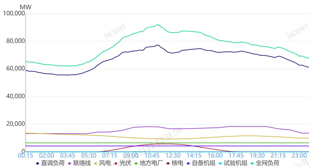
图1 10月9日负荷及电源出力预测情况
