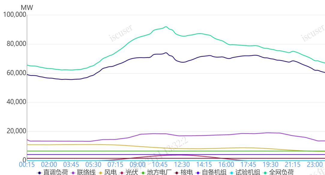
图 1 10月10日负荷及电源出力预测情况
