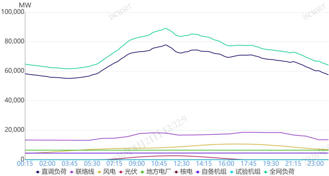
图 1 10月12日负荷及电源出力预测情况
