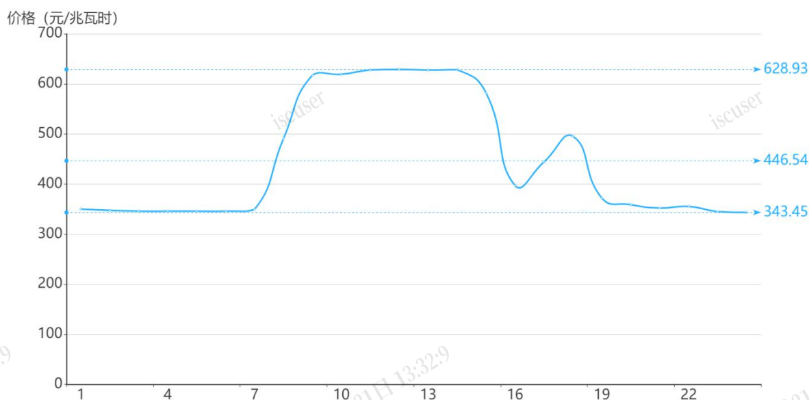
图 2 10 月 12 日日前市场用电侧价格
