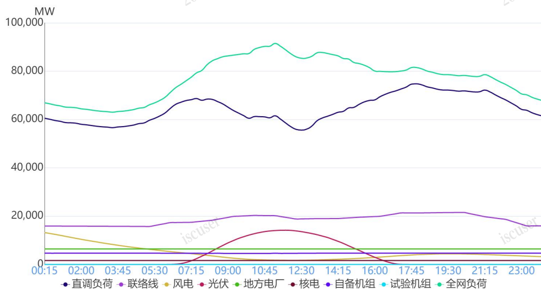
图 1 10月30日负荷及电源出力预测情况
