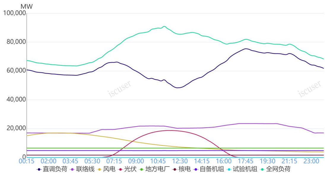
图 1 11 月 2 日负荷及电源出力预测情况
