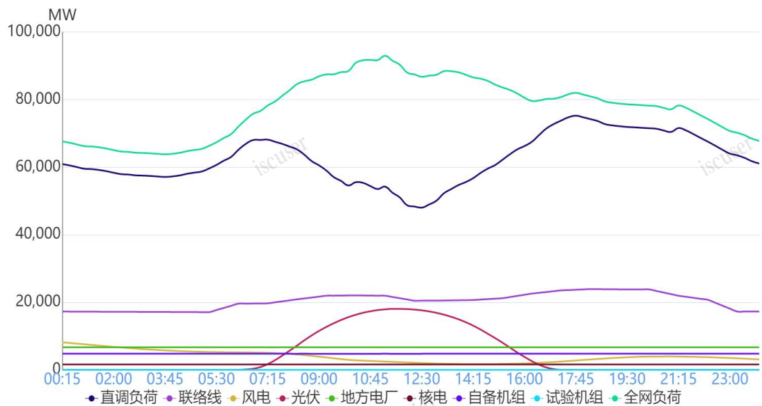
图 1 11 月 5 日负荷及电源出力预测情况
