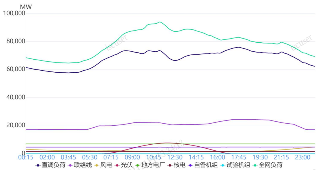
图 1 11月8日负荷及电源出力预测情况
