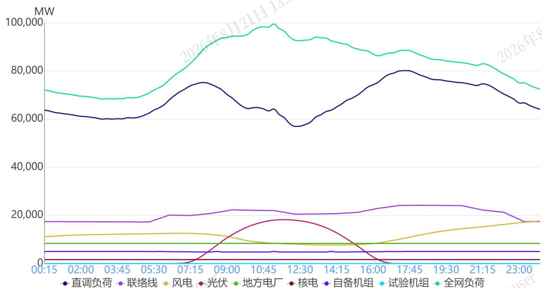
图 1 11月26日负荷及电源出力预测情况
