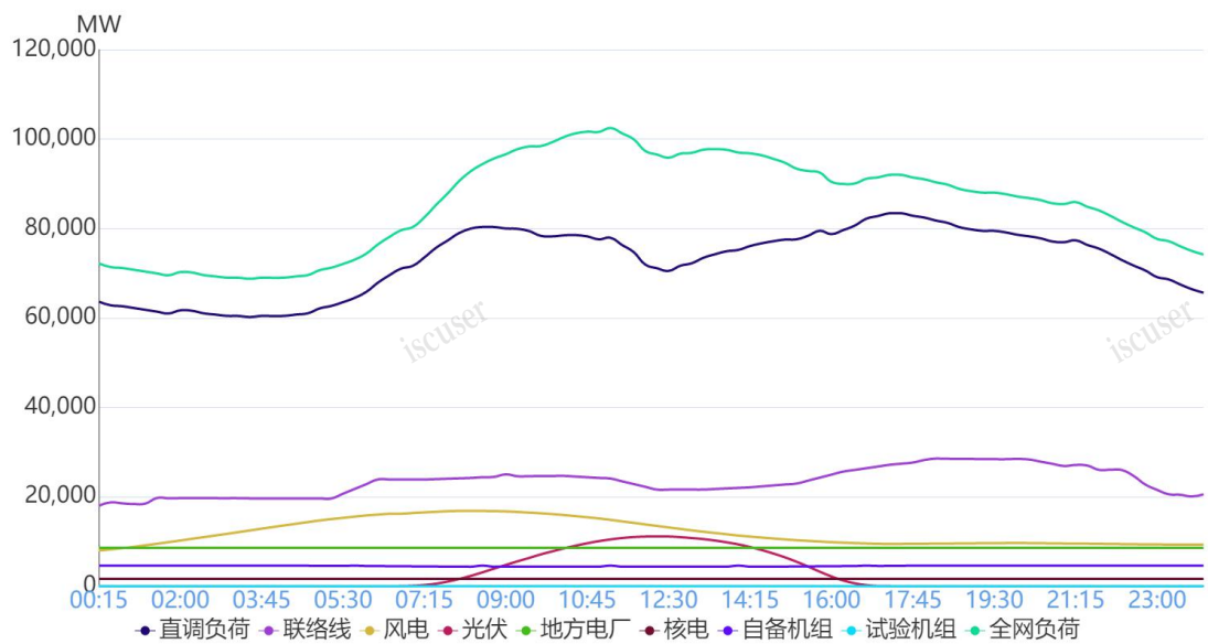
图 1 12 月 2 日负荷及电源出力预测情况
