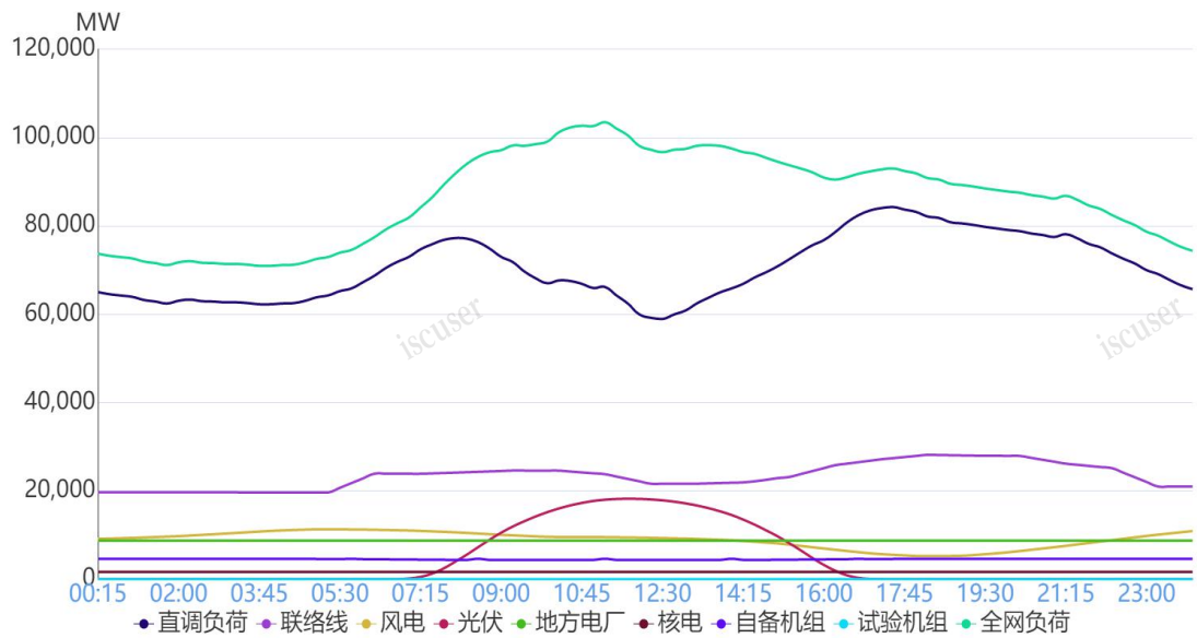
图 1 12 月 3 日负荷及电源出力预测情况
