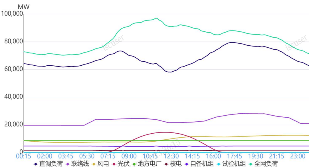
图 1 12月7日负荷及电源出力预测情况
