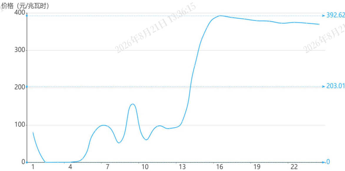
图 3 12 月 6 日实时市场用电侧价格
