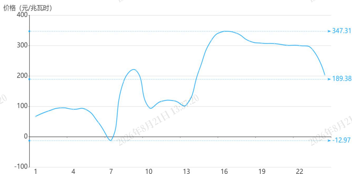
图2 12月19日日前市场用电侧价格
