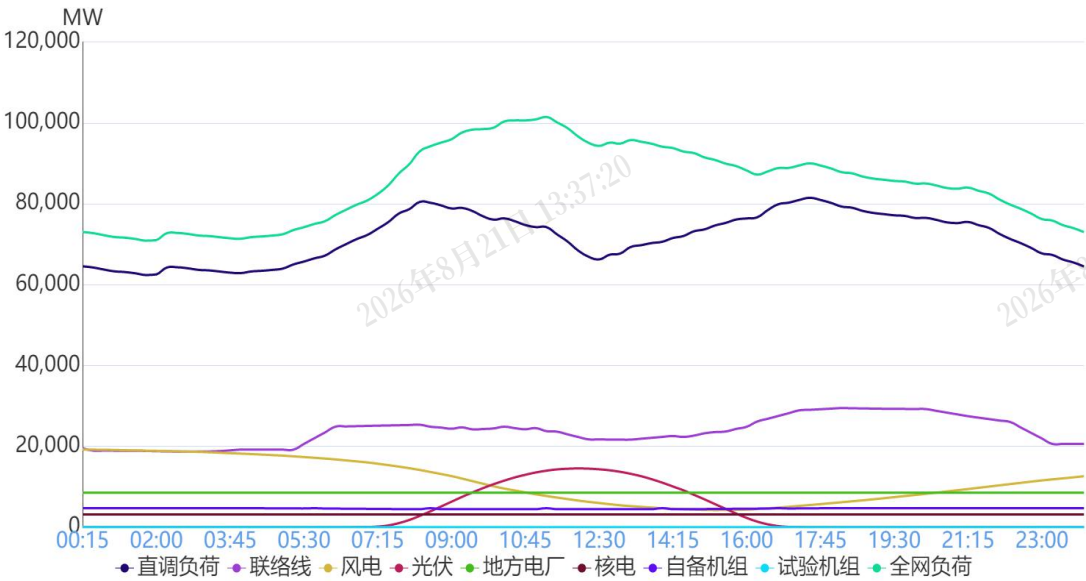
图1 12月19日负荷及电源出力预测情况
