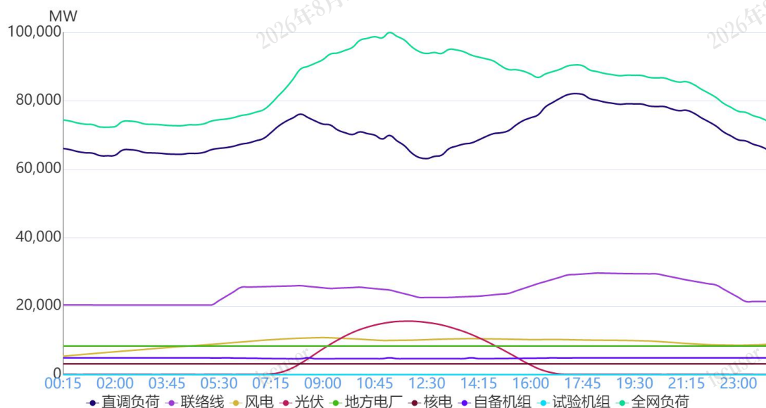
图 2 12月28日负荷及电源出力预测情况
