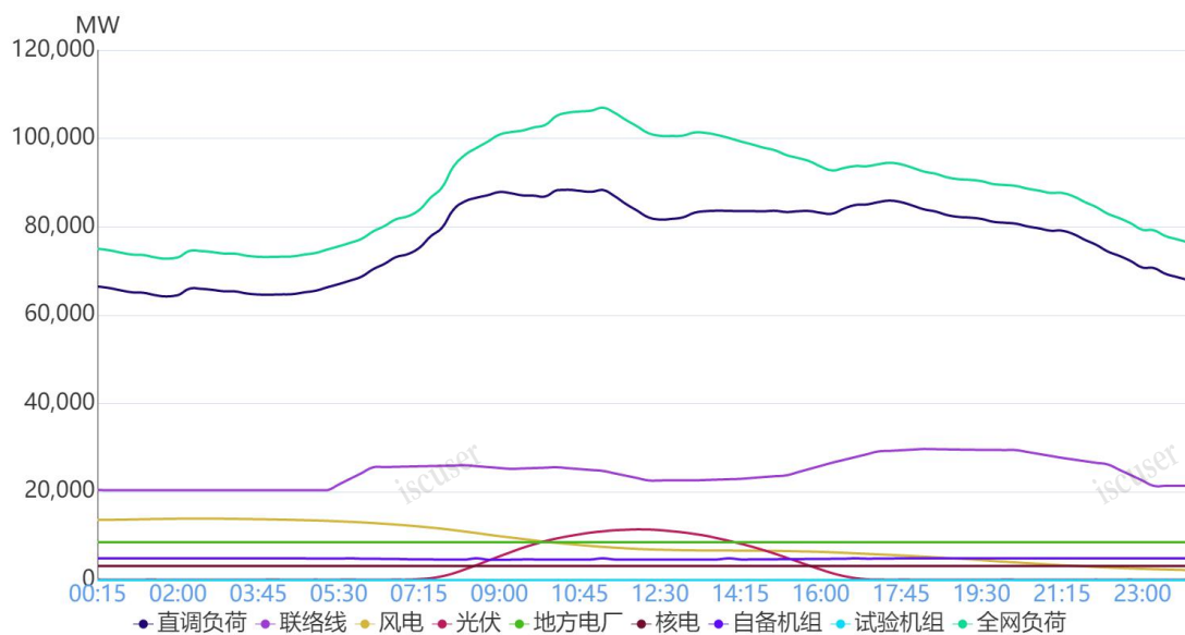
图 1 12月31日负荷及电源出力预测情况
