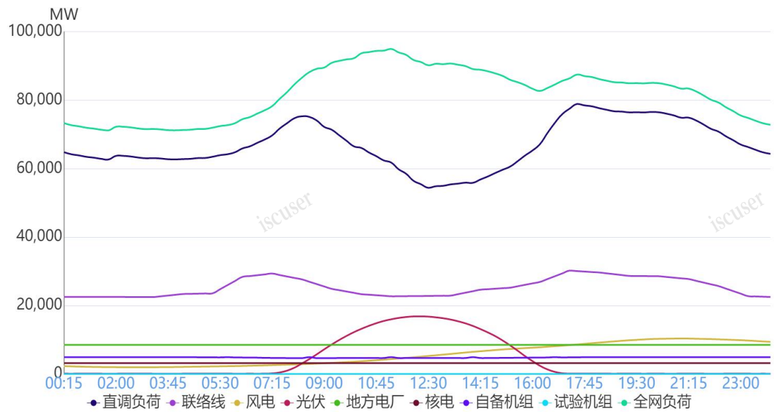
图 1 1 月 1 日负荷及电源出力预测情况
