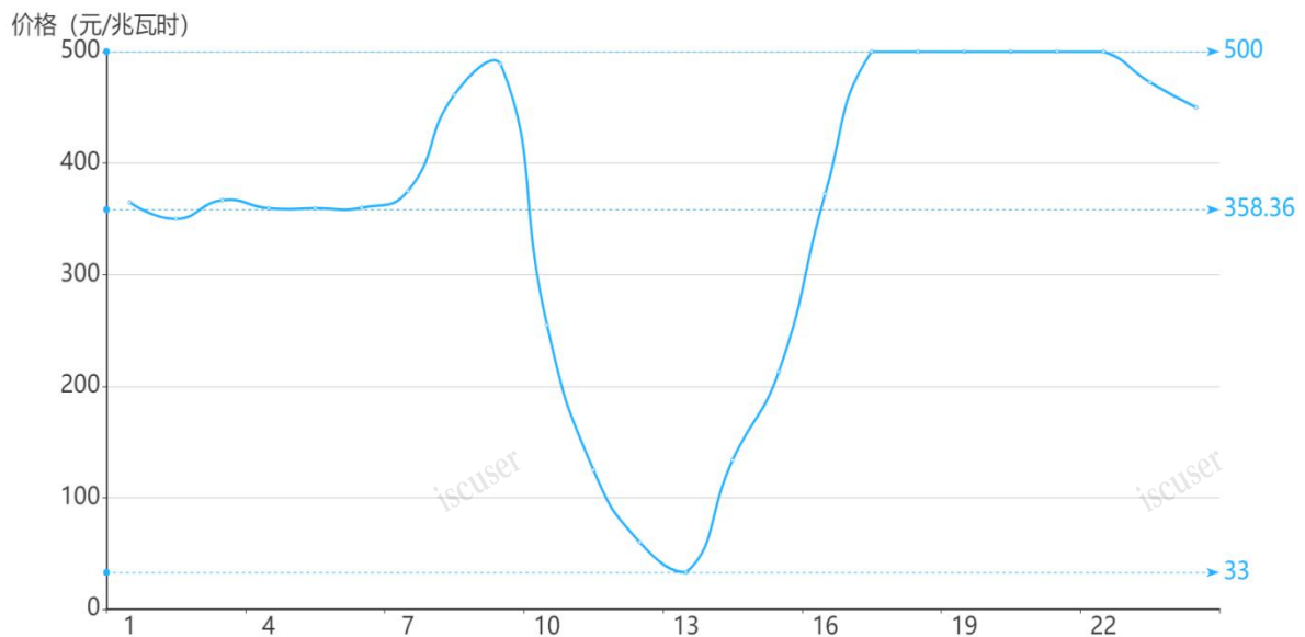
图2 1月3日日前市场用电侧价格
